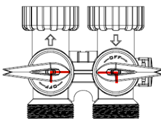
Положение байпас
